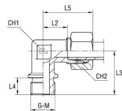
B3-leikkuurengasliitoksella
