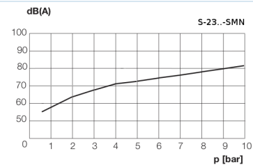
Geluidsniveau
