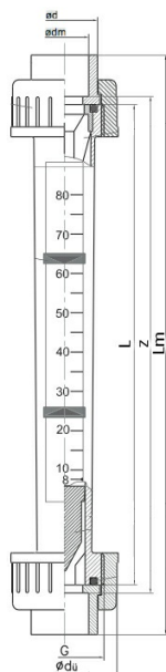
(1)...Hegeszthető csomos csavarzat, (2)...Menetes hüvelyes csatlakozó idom
