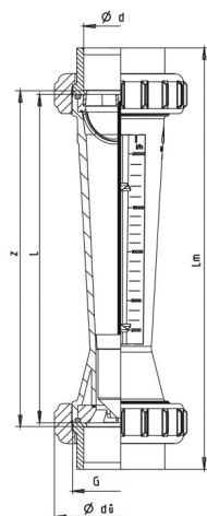
(1)...Hegeszthető csónkos csavarzat, (2)...Menetes hüvelyes csatlakozó idom
