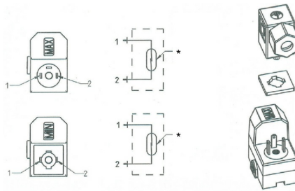
*Liitäntäjärjestys Reed-kytkin
