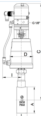
I/P-positioneringsregulator Type 8047
