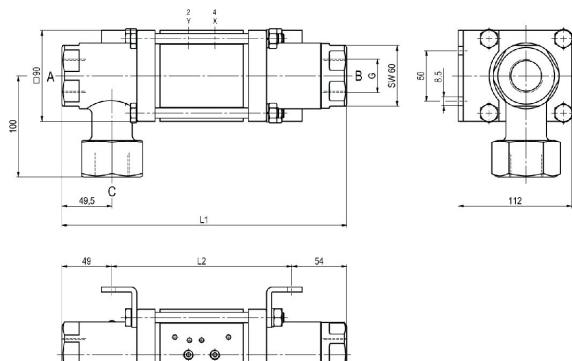
CVTE3-25 Funksjon NC
