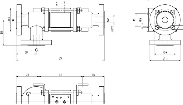
CVFE3-20 Funzione NO
