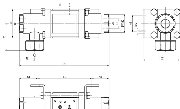
CVTE3-20 Funzione NC
