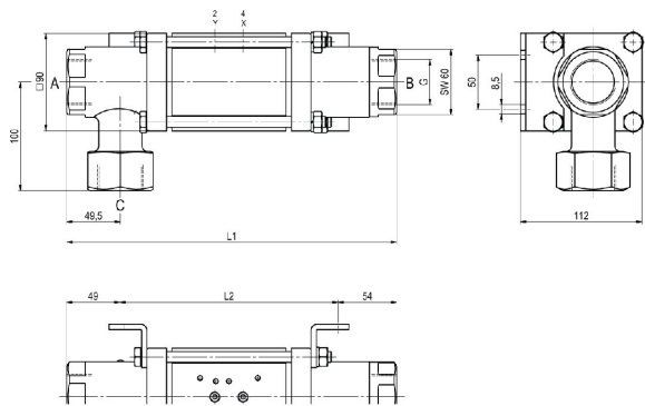
CVTE3-32 Funktion NC
