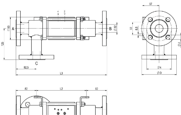
CVFE3-32 Funktion NO
