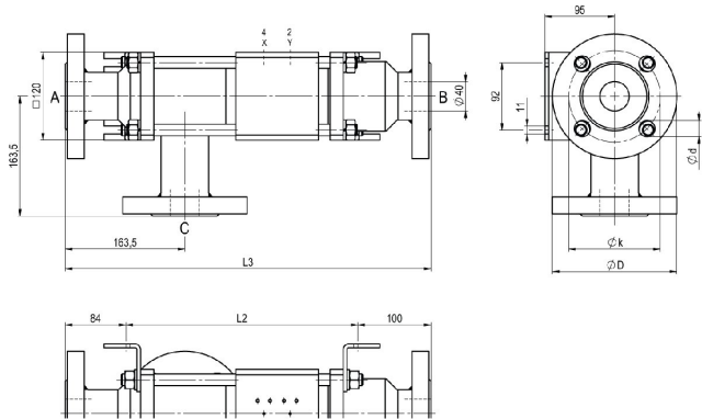
CVTE3-40 Funksjon NC
