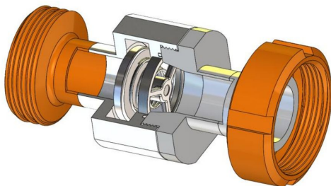
Mit montierten Gewindestutzen With mounted thread connectors
