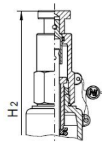
Κεφαλή στεγανό ως προς το αέριο με κουμπτί εξαέρωσης
