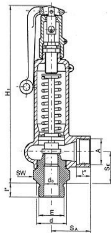
Tête Levier de purge étanche au gaz
