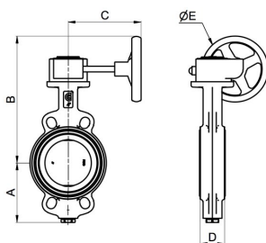
Mellemflangeudførelse
