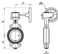
Međuprostavna izvedba priрубnice
