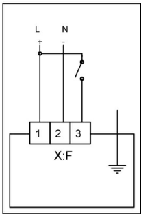
Commande 2 points
