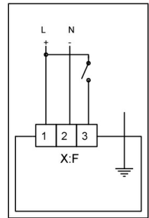
2-punktsstyring
