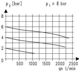
Wykres przepływu
