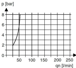
Oljeapparatets aktiveringsgrense
