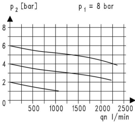
Diagramme de débit
