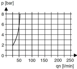
Seuil de déclenchement du lubrificateur
