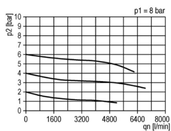
Strømningsdiagramm
