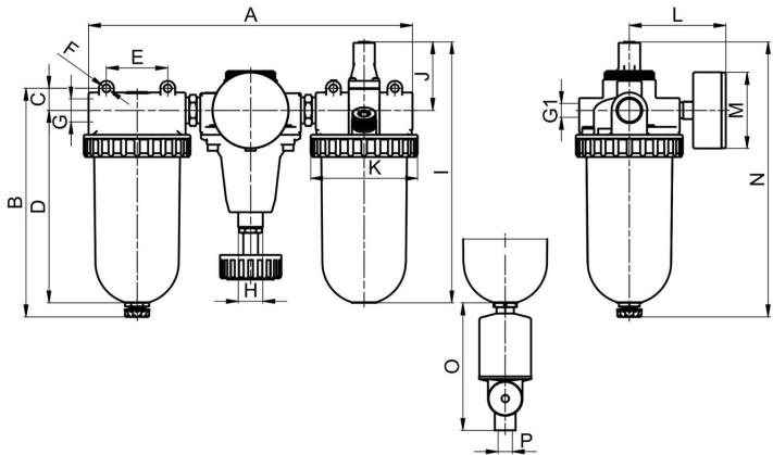
purgeur automatique
