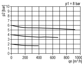
Doorstroomdiagramma
