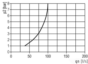
Olievernevelaar-inschakeldrempel
