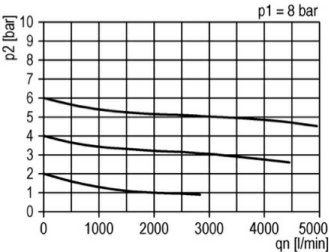
Strømningsdiagramm
