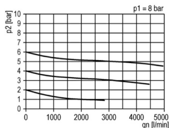
Dijagram protoka
