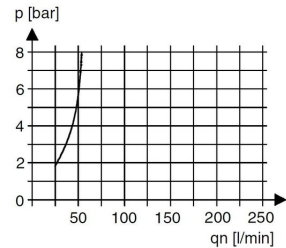
Olieforstøverens aktiveringsgrænse
