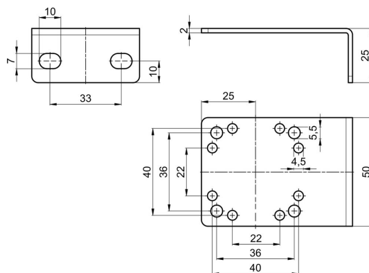
Staffa di fissaggio Tipo MMB-RE6263-01
