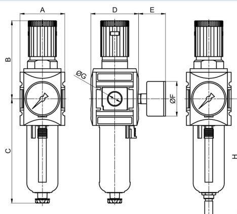
halvautomatisk aftapningsventil
