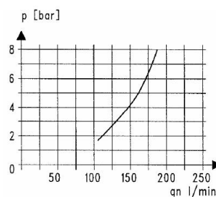
Olieforstøverens aktiveringsgrænse
