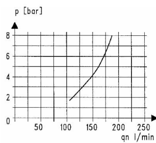
Olievernevelaar-inschakeldrempel
