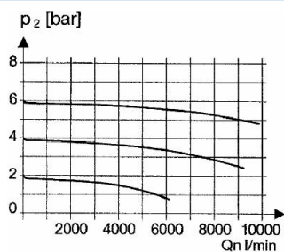
Διάγραμμα ροής
