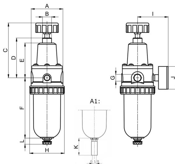
A1: automaattinen tyhjennysventtiili
