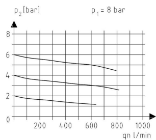
Virtauskaavio
