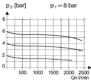
Strømningsdiagramm
