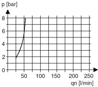
Oljeapparatets aktiveringsgrense
