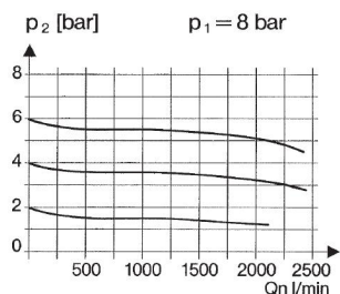
Virtauskaavio
