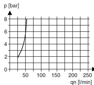
Öljysumuttimen toimintaraja
