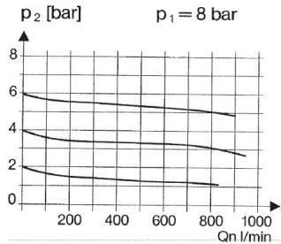
Diagramma di portata
