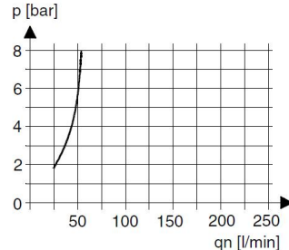
Soglia di intervento dell'oliatore
