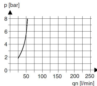
Öljysumuttimen toimintaraja
