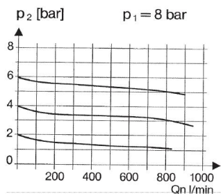
Virtauskaavio
