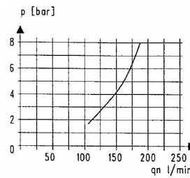
Öljysumuttimen toimintaraja
