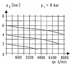
Virtauskaavio
