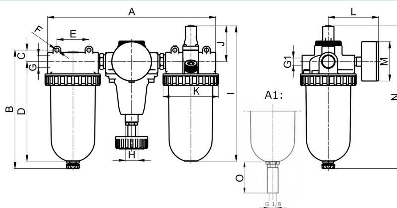
A1: automatisk tappeventil
