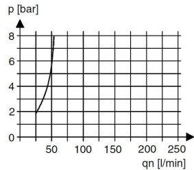
Olieforstøverens aktiveringsgrænse
