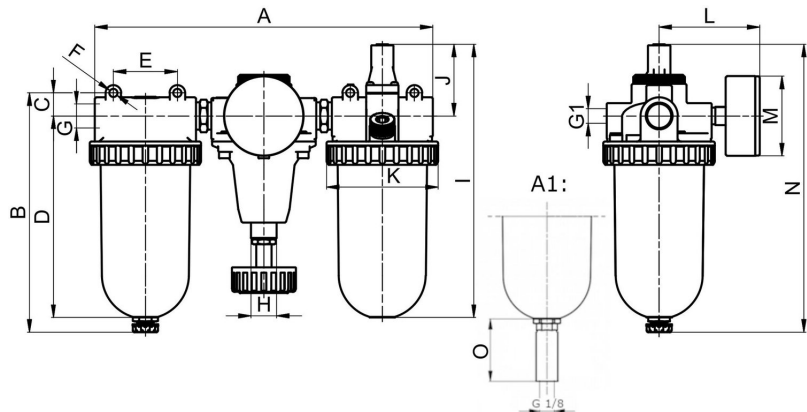
A1: automatisch aftapventiel
