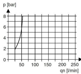
Olievernevelaar-inschakeldrempel
