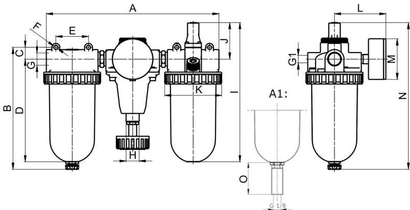
A1: automatisches Ablassventil
