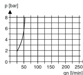
Olieforstøverens aktiveringsgrænse
