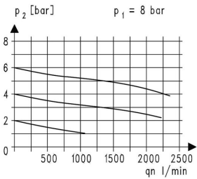
Průtokový diagramm
