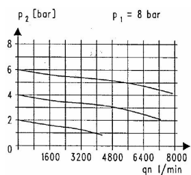
Diagramă de debit
