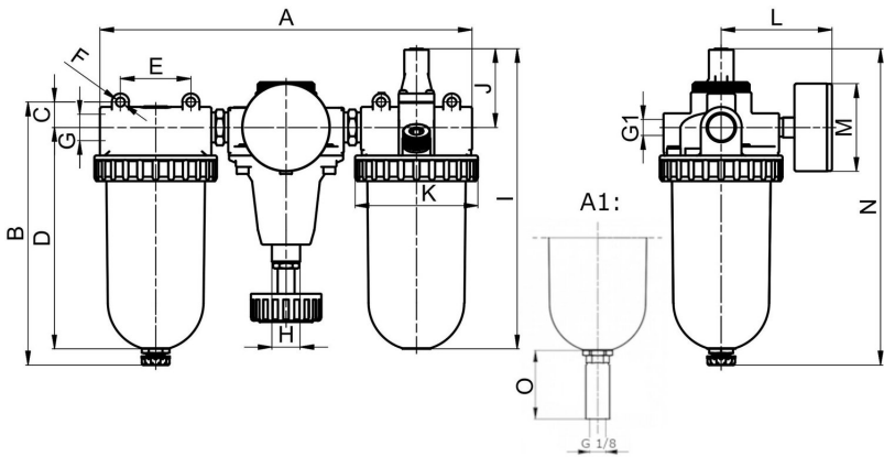
A1: purgeur automatique
