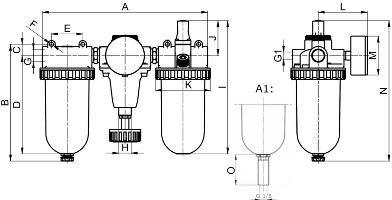
A1: automatyczny zawór spustowy
