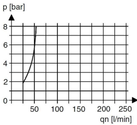
Oljeapparatets aktiveringsgrense
