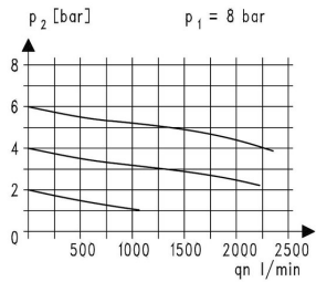
Diagramme de débit
