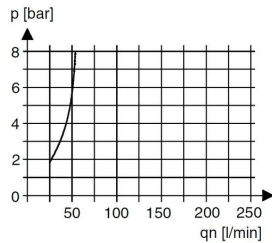
Olieforstøverens aktiveringsgrænse
