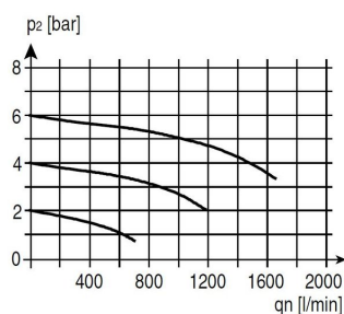
Virtauskaavio
