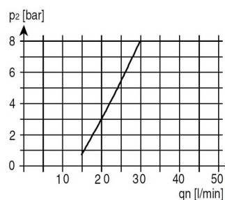
Öljysumuttimen toimintaraja
